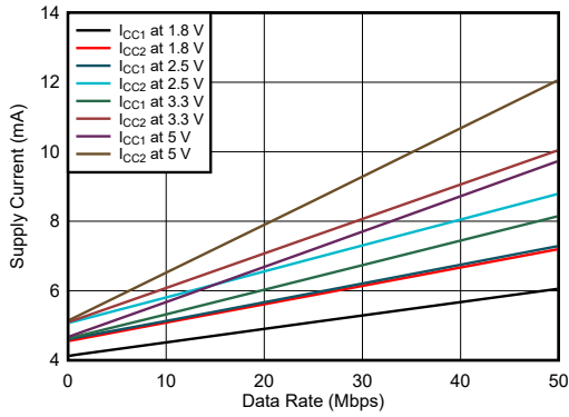
图 6-9. ISO6763 电源电流与数据速率间的关系 (具有 15pF 负载)
