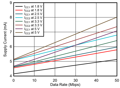
图 6-10. ISO6763 电源电流与数据速率间的关系 (无负载)
