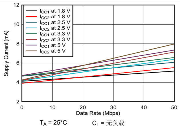
图 6-8. ISO6762 电源电流与数据速率间的关系 (无负载)
