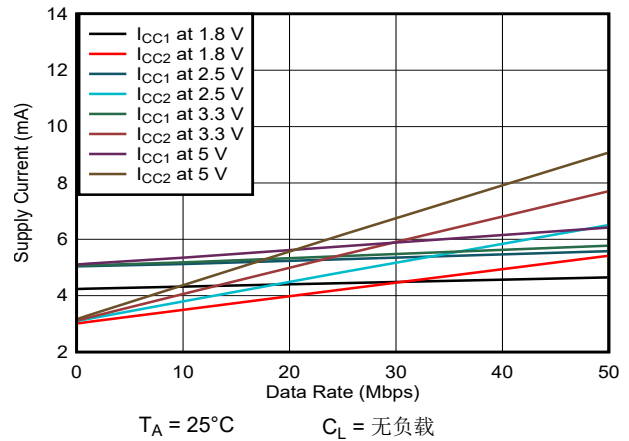
图 6-4. ISO6760 电源电流与数据速率间的关系 (无负载)
