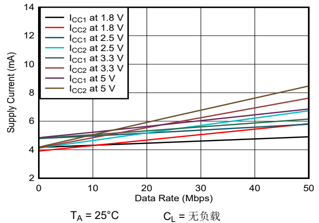
图 6-6. ISO6761 电源电流与数据速率间的关系 (无负载)
