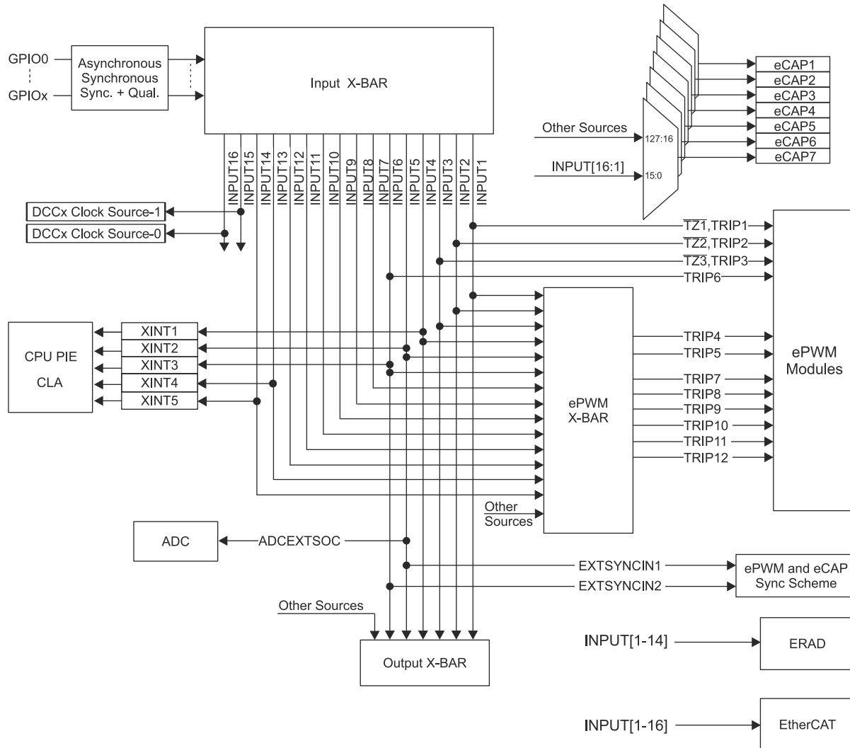
图 6-7. Input X-BAR
