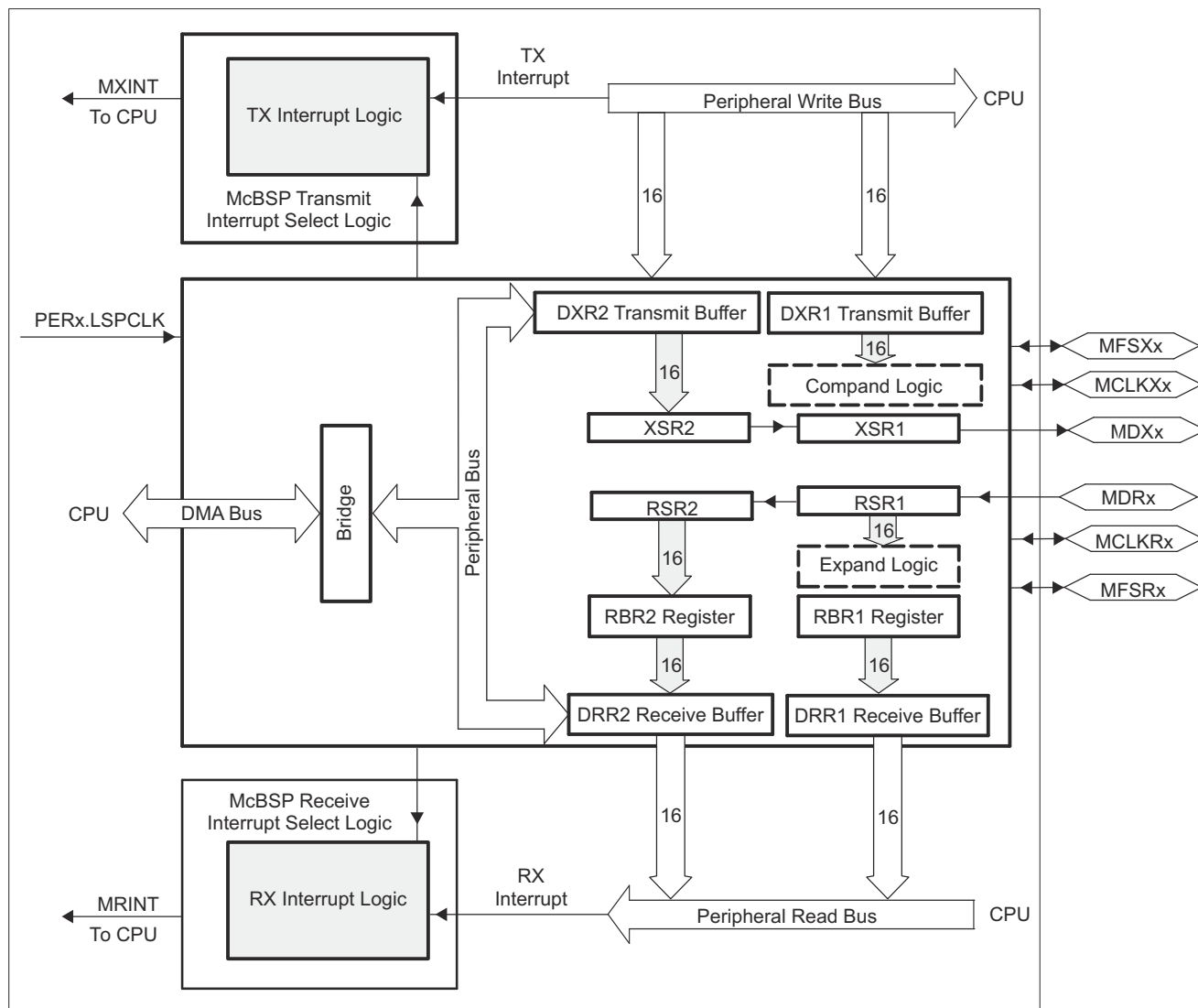
图 7-68. McBSP Block Diagram
