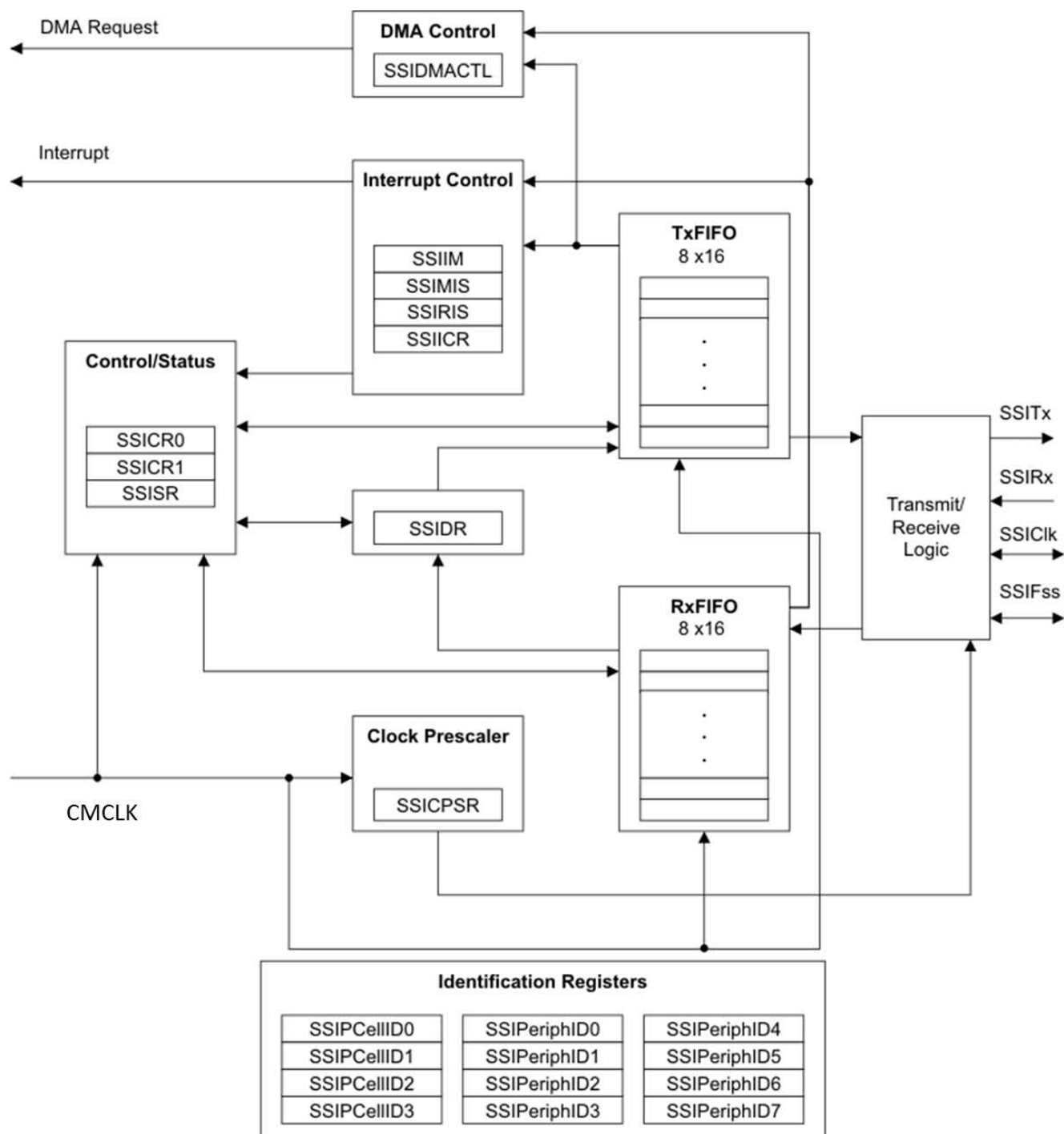
图 7-99. SSI Block Diagram
