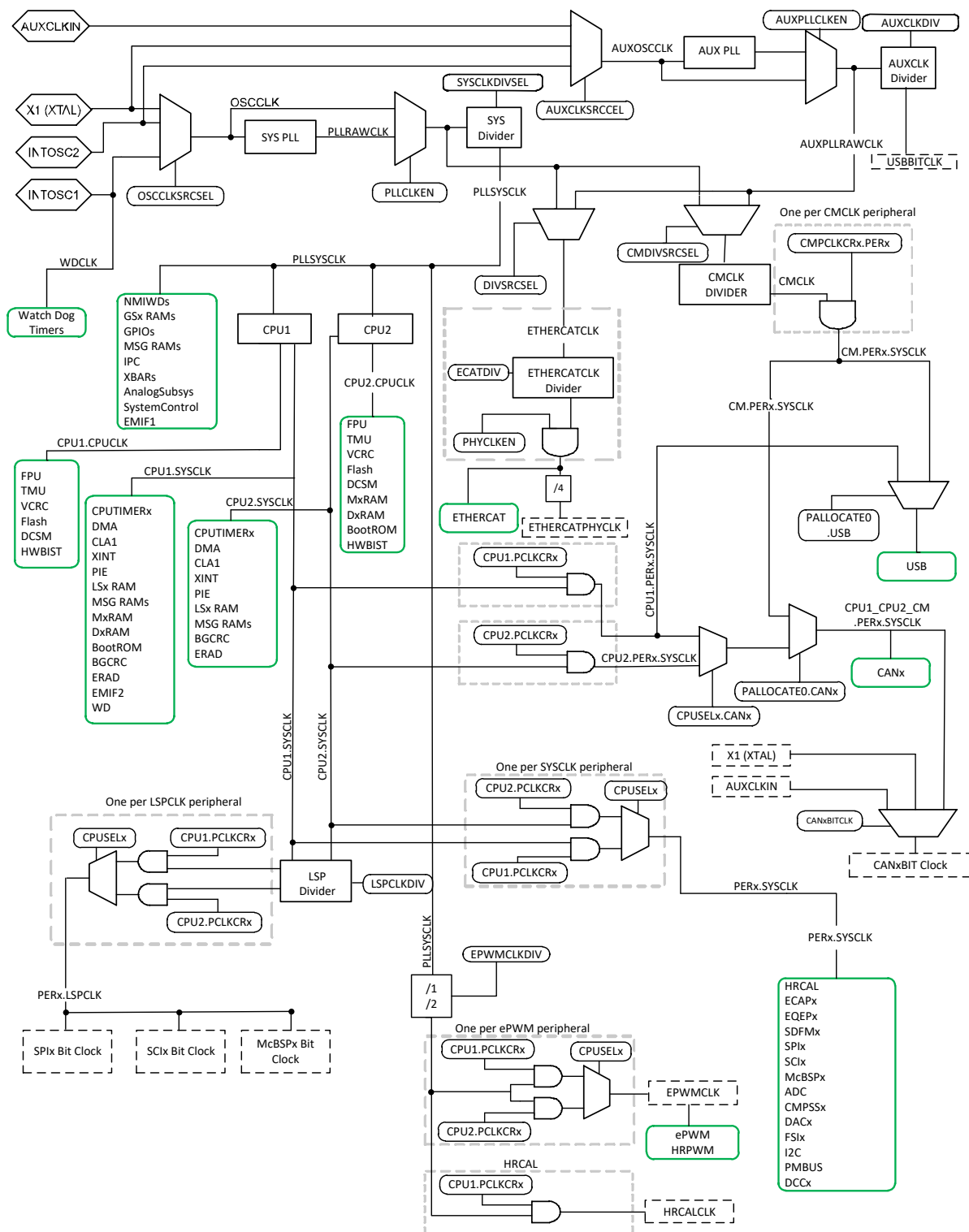
图 7-7. Clocking System
