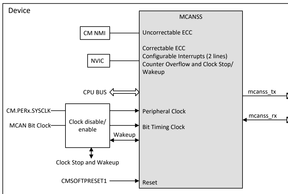
图 7-89. MCAN Module Overview
