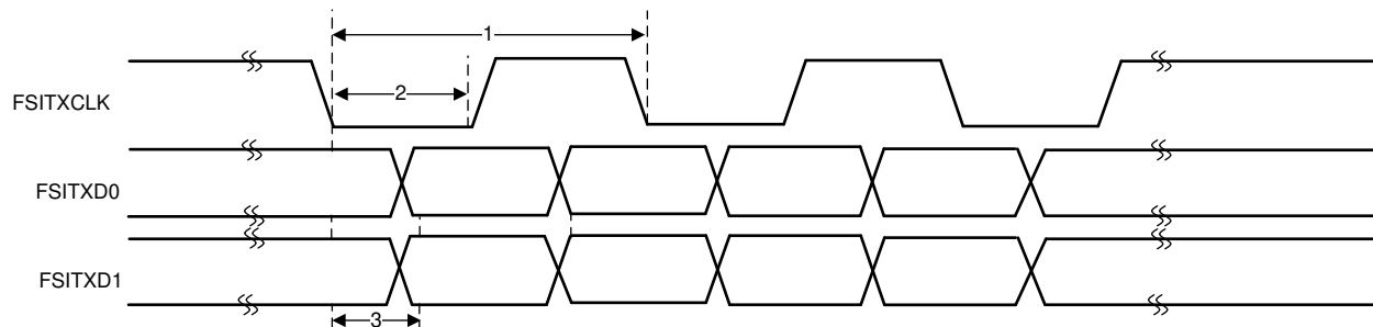
图 7-61. FSITX Timings
