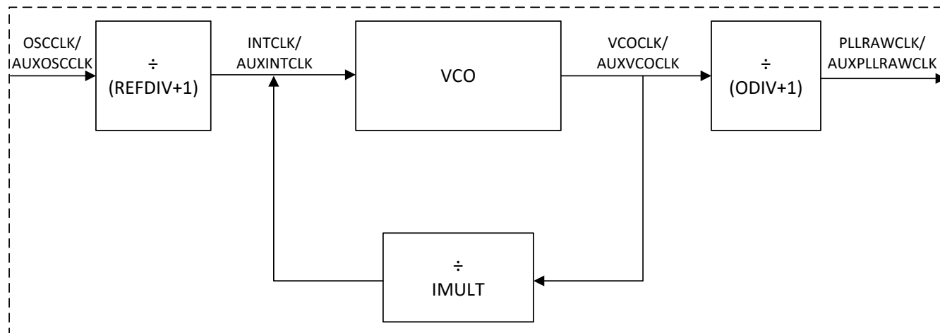
图 7-8. SYSPLL/AUXPLL
