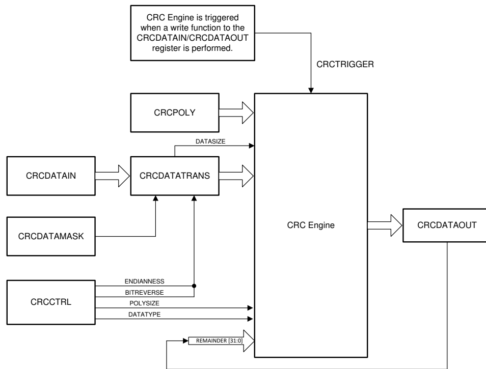
图 8-11. GCRC Block Diagram
