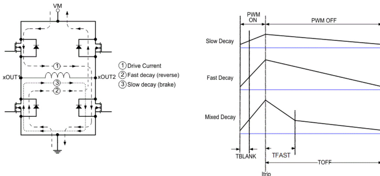
图 7-6. Decay Modes
