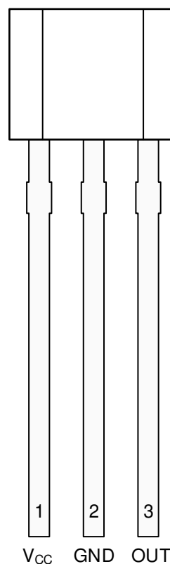
图 5-2. LPG 封装 3 引脚 TO-92 顶视图
