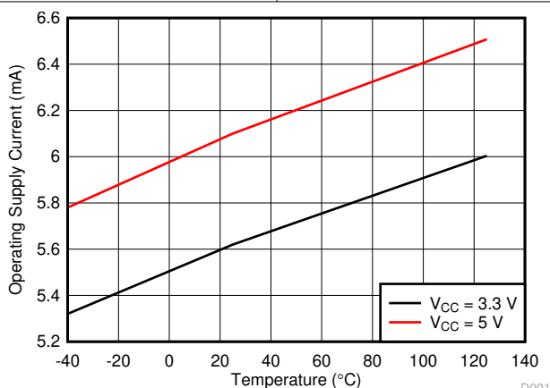
图 6-13. 工作电源电流与温度之间的关系
