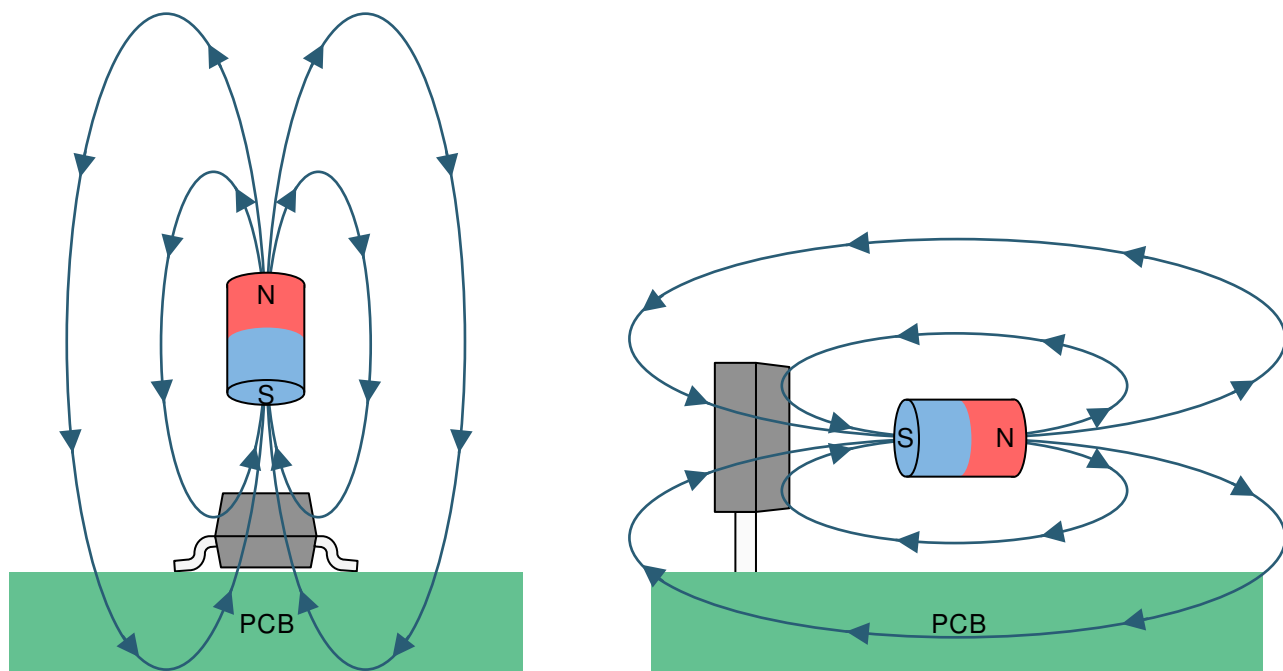
图 7-2. 正 B 的磁通方向
