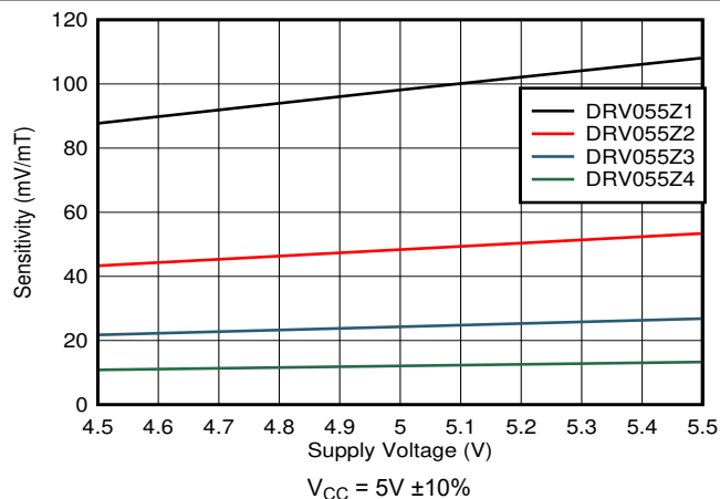
图 6-12. 灵敏度与电源电压之间的关系
