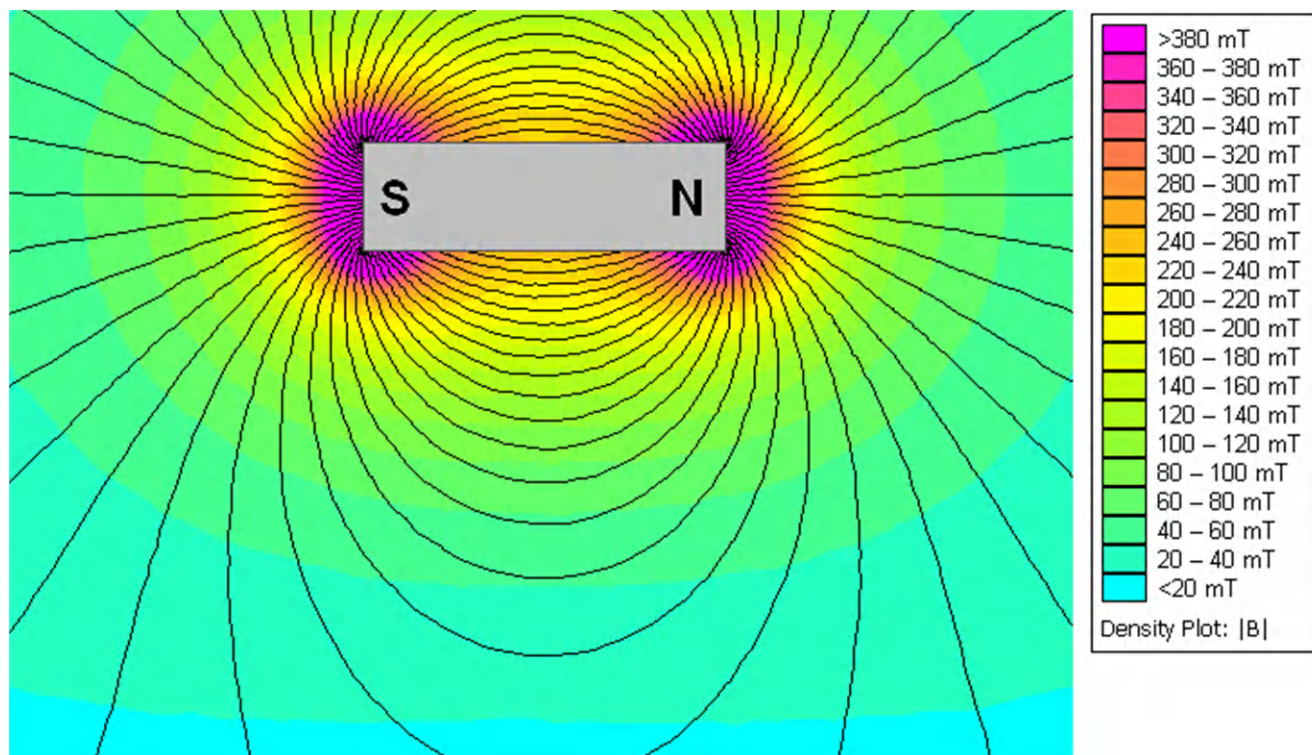
图 8-3. 仿真磁通
