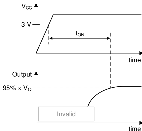
图 7-4. t_{ON} 定义
