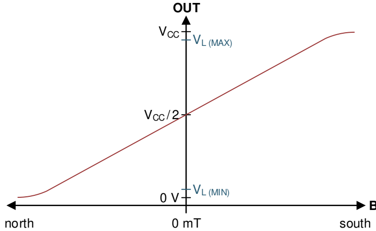
图 7-3. 磁响应
