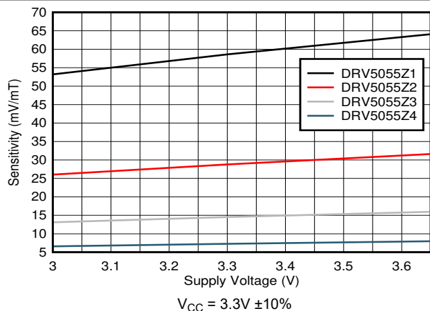
图 6-11. 灵敏度与电源电压之间的关系
