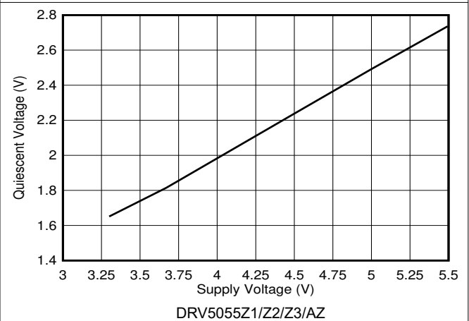
图 6-4. 静态电压与电源电压之间的关系
