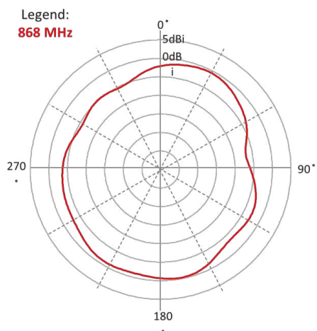
Elevation 1
