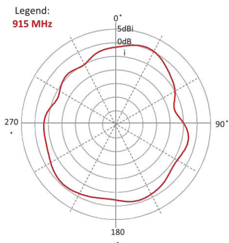
Elevation 1
