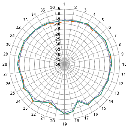
XZ-Plane Gain
