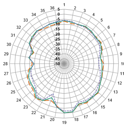
YZ-Plane Gain
