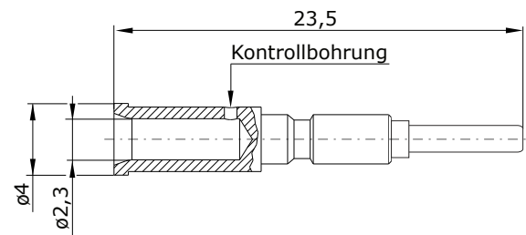
Hauptabmessungen Kontaktstift
