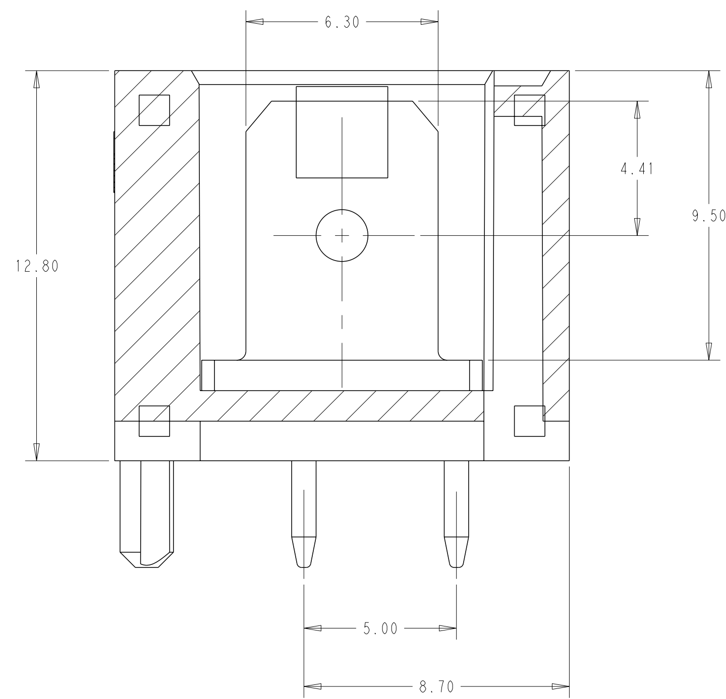
SECTION A-A
