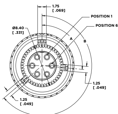
Receptacle Key
