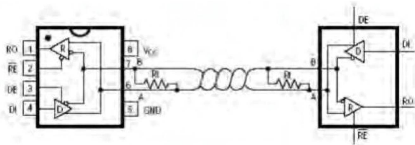
图2 产品应用示意图
