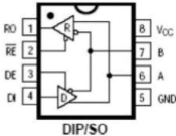
图1封装图
