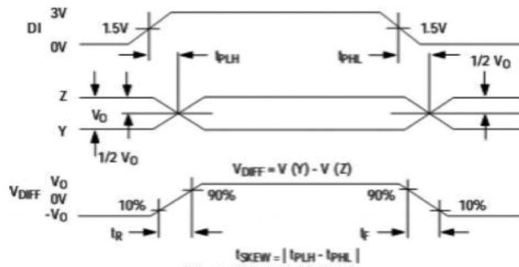
图 8 驱动传输延时
