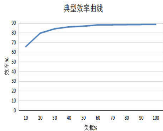
12V 输出典型效率曲线图
