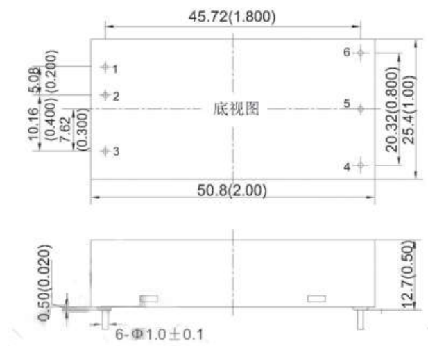
T_LD-30WR3Q 尺寸图
