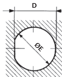
Type 7 jam nut receptacle
