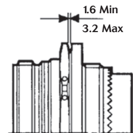
Type 7 jam nut receptacle
