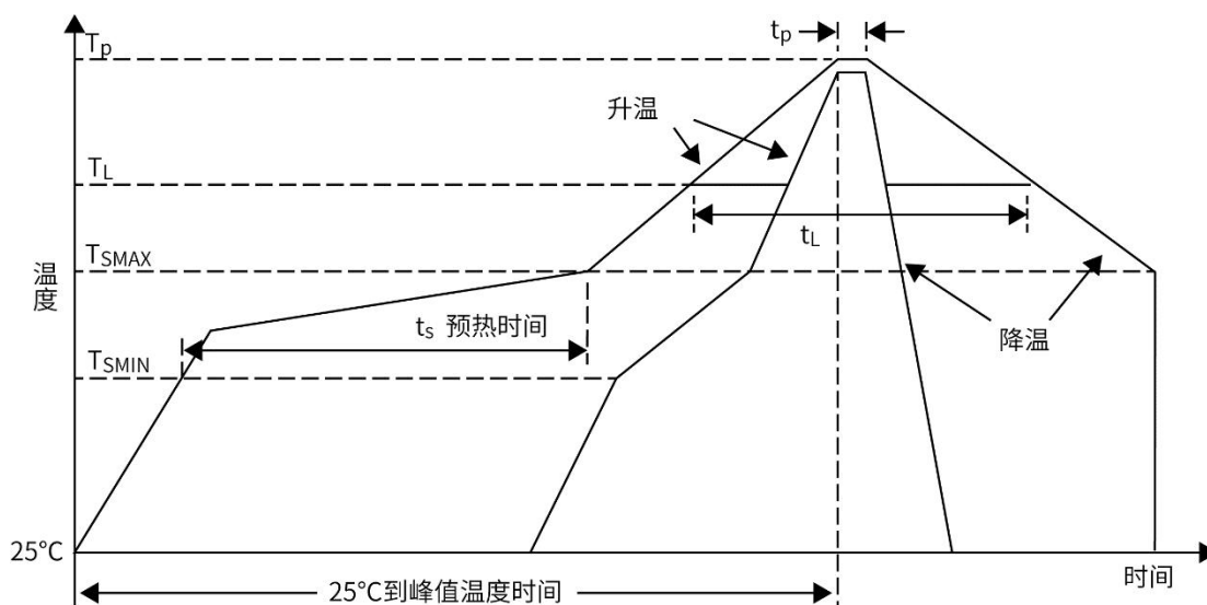
图 10. 推荐无铅焊锡回流温度曲线分布图
