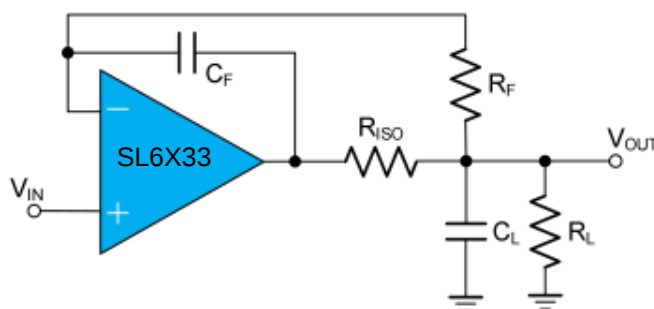
图 3 直接驱动容性负载且具有高的 DC 精度
