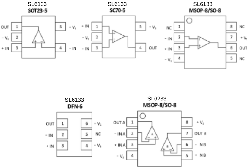
图 1 管脚分布
