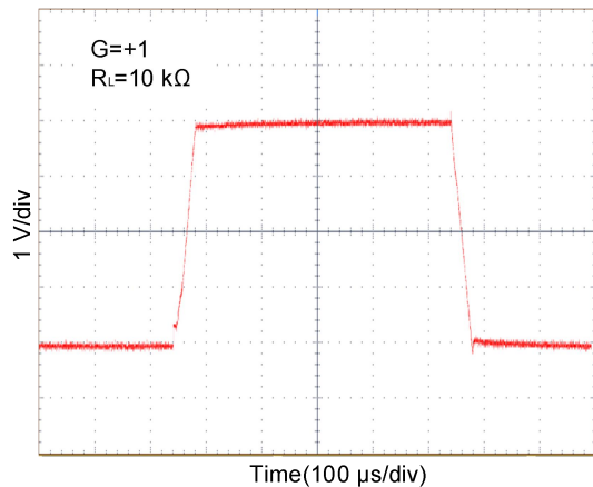
大信号阶跃响应+5V
