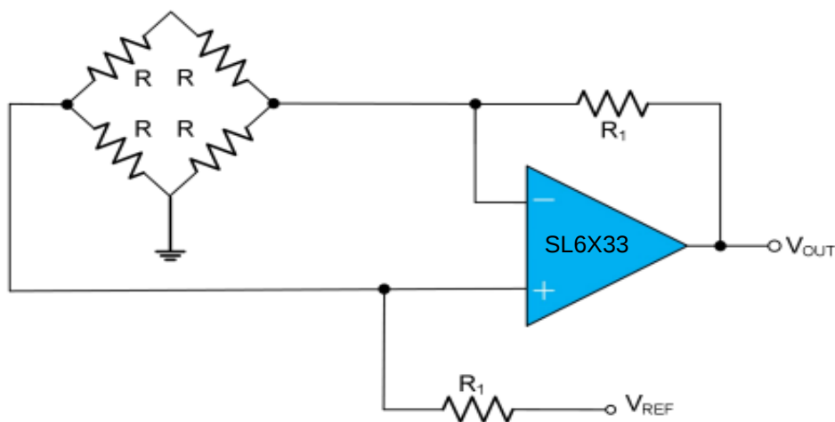
图 5 桥式放大器
