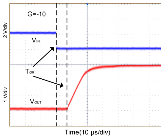
负过载恢复
