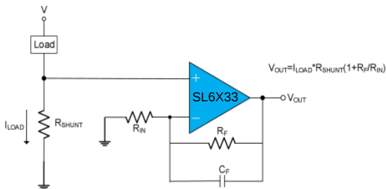
图 4 低侧电流采样电路
