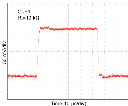
小信号阶跃响应+5V
