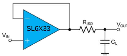
图 2 间接重的容性过载
