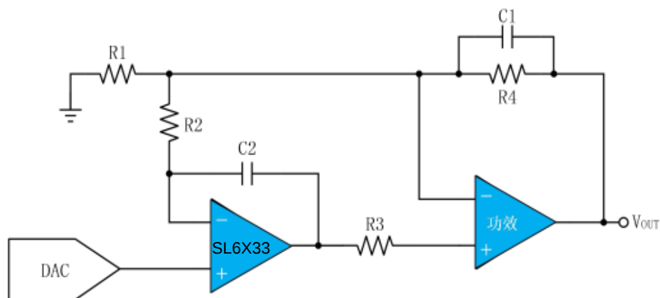
图 6 可编程电压源
