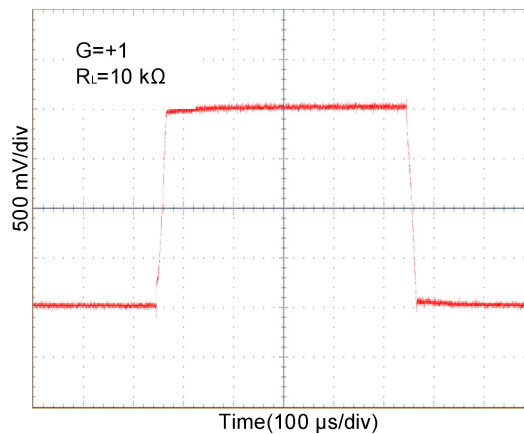
大信号阶跃响应+2.7V
