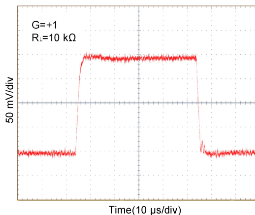
小信号阶跃响应+2.7V
