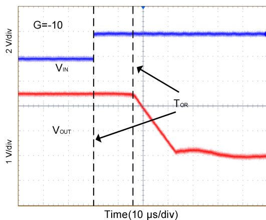
正过载恢复
