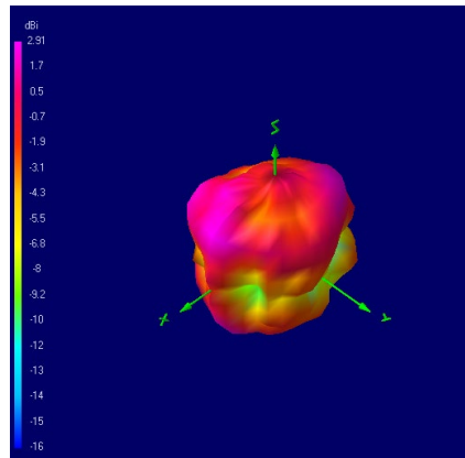
2437 MHz
