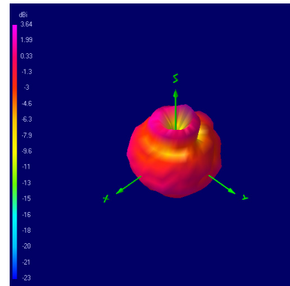
6060 MHz
