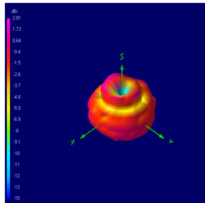
6180 MHz
