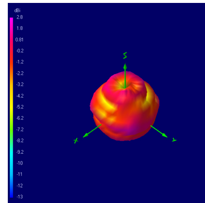
6520 MHz
