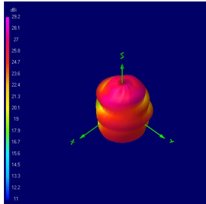
1227.6 MHz
