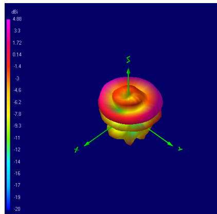
5512 MHz
