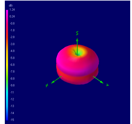
3432 MHz
