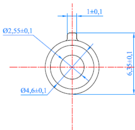
侧视图
