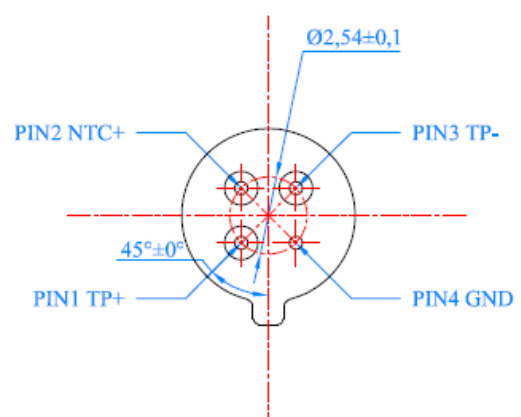
电气连接
