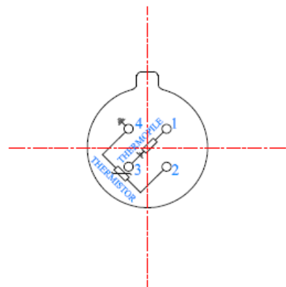
电气连接
