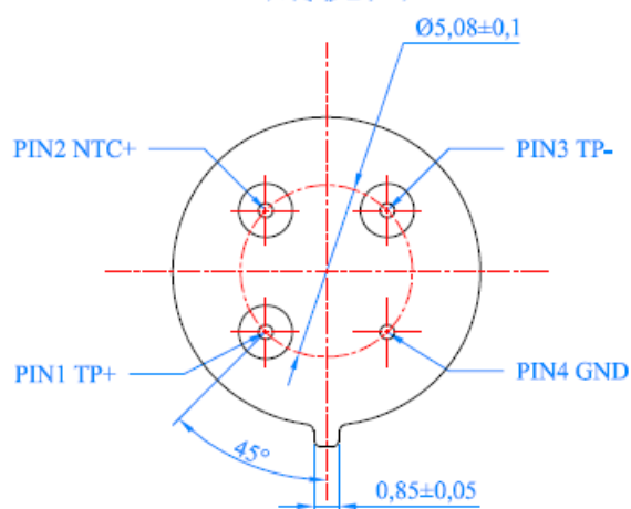
底视图
