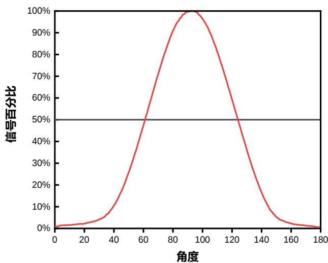
SY-TP-36BPDG视场角
