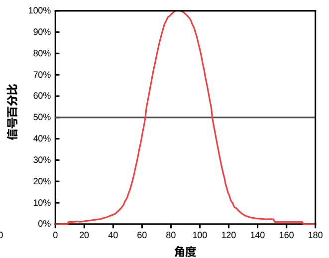
SY-TP-36BPDG-A视场角
