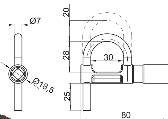
PADLOCK SN 4.KDZN.001
