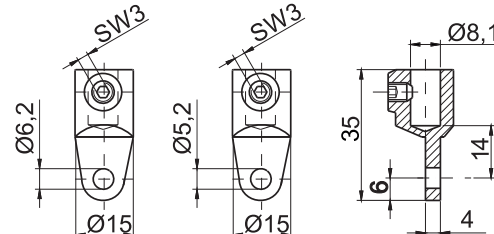
ROD HOLDER
