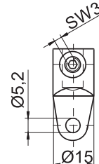
ROD HOLDER
