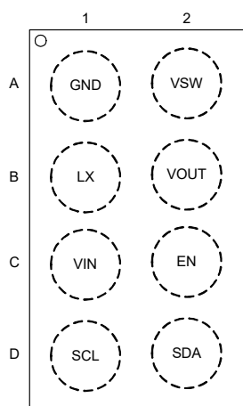
8 Bump WLCSP
