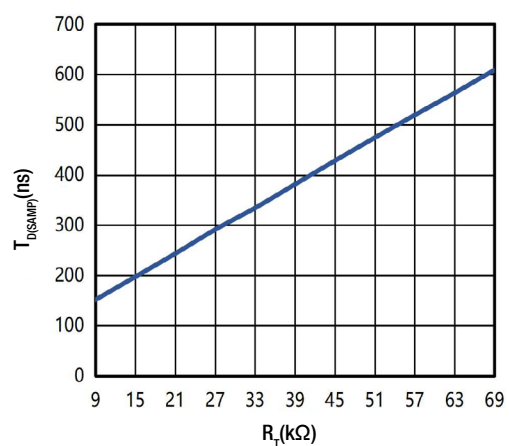
Fig. 12. T_{D(SAMP)} vs R_T
