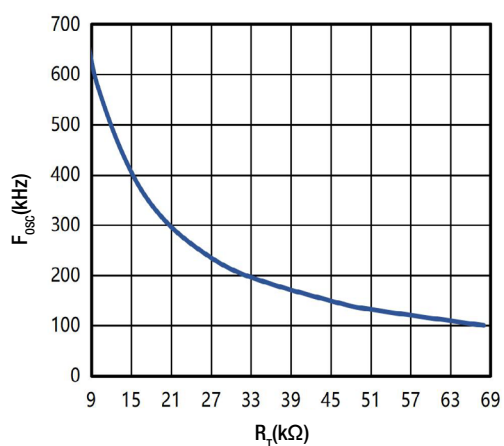
Fig. 11. F_{osc} vs R_T
