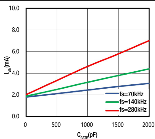
Fig. 10. I_{VIN} vs C_{GATE}
