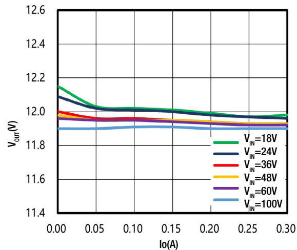
Fig. 23 Vout vs Io
