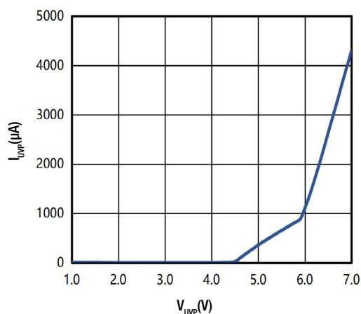
Fig. 7. I_{UVP} vs V_{UVP}
