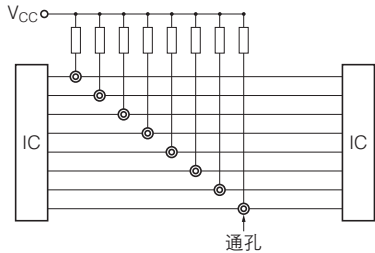
上拉电阻
