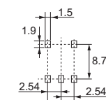
Actual Mounting Pad Dimensions
