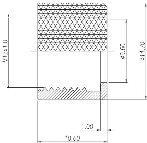
NUT
