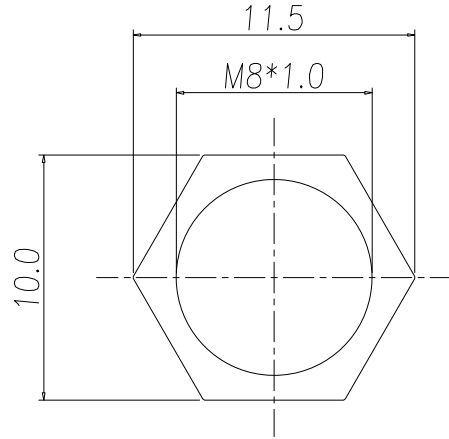
NUT
