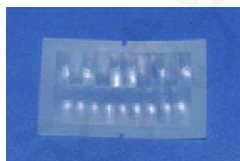
型号: 7805-1 尺寸: 56.7*35.8 焦距: 22mm 感应角度: 100° 感应距离: 10m
