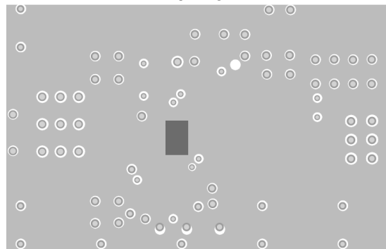
Inner Layer 1
