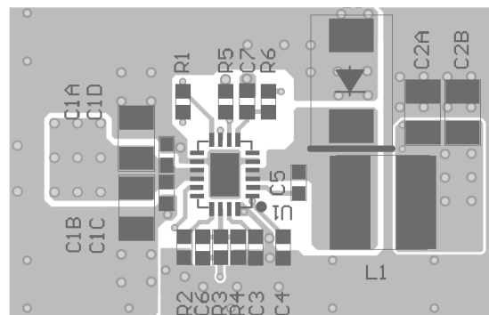
Top Layer
