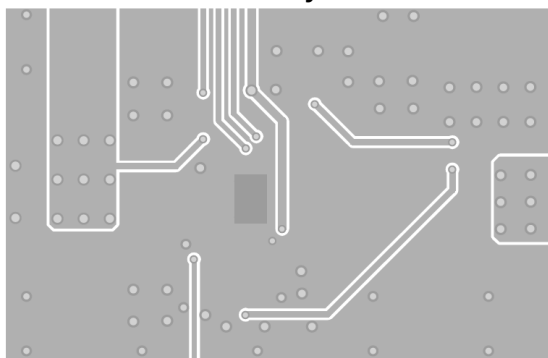
Inner Layer 2
