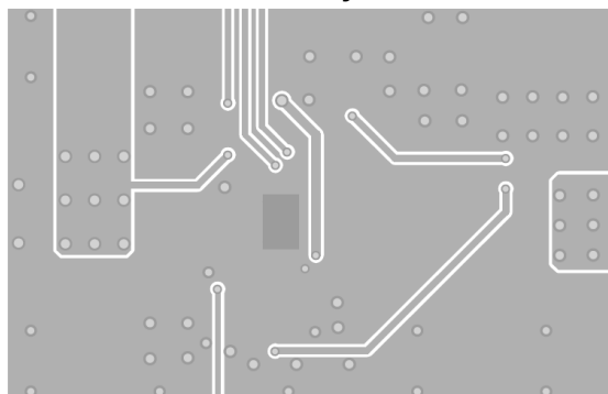
Bottom Layer
