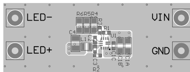
Top Layer
