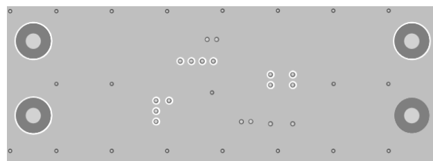
Bottom Layer
