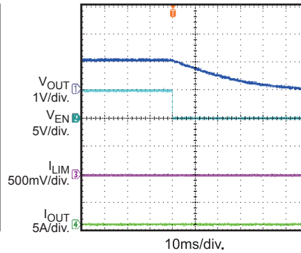
Enable Shutdown
