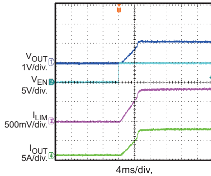
Enable Startup
