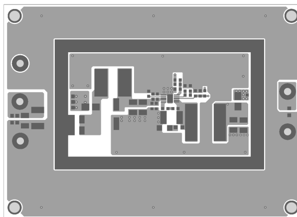
Figure 2—Top Layer
