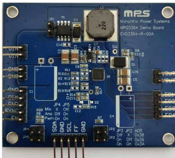
Top Layer
