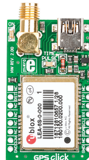
GPS click™
