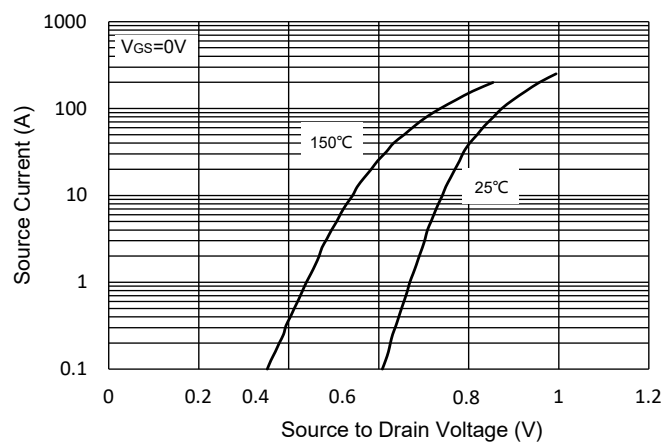
Fig.9 - I_S - V_{SD}
