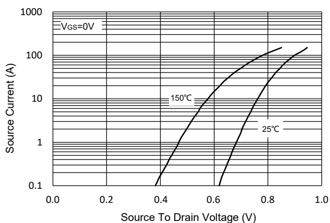
Fig.9 - I_S - V_{SD}
