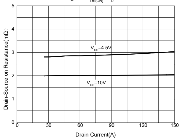
Fig. 4 - R_{DS(ON)} - I_D
