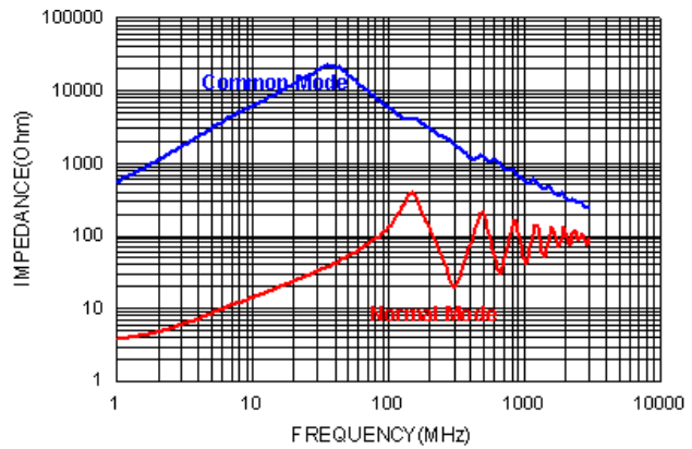
ACT4532L-101-2P-TF
