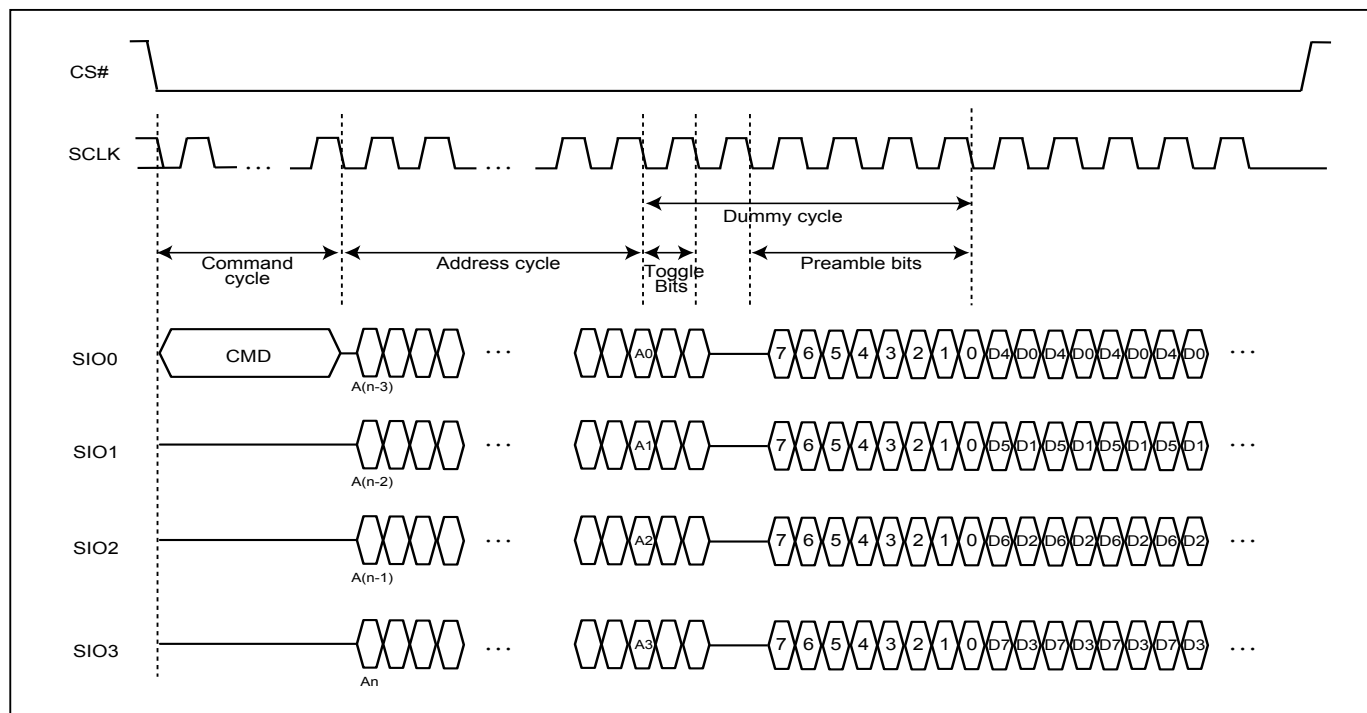
Figure 55. DTR4IO (DC=6)
