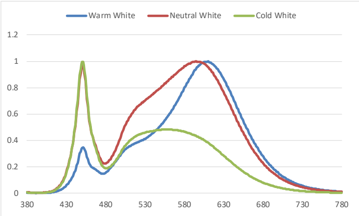
Color Spectrum ( CRI≥80Tc=25°C )
