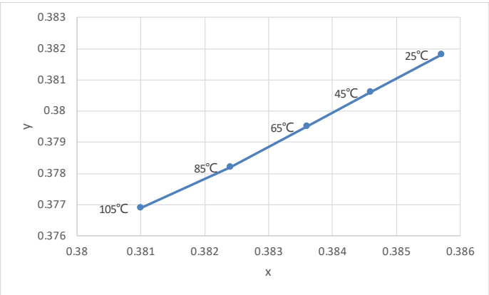
Case Temperature VS. CIE X, Y SHIFT
