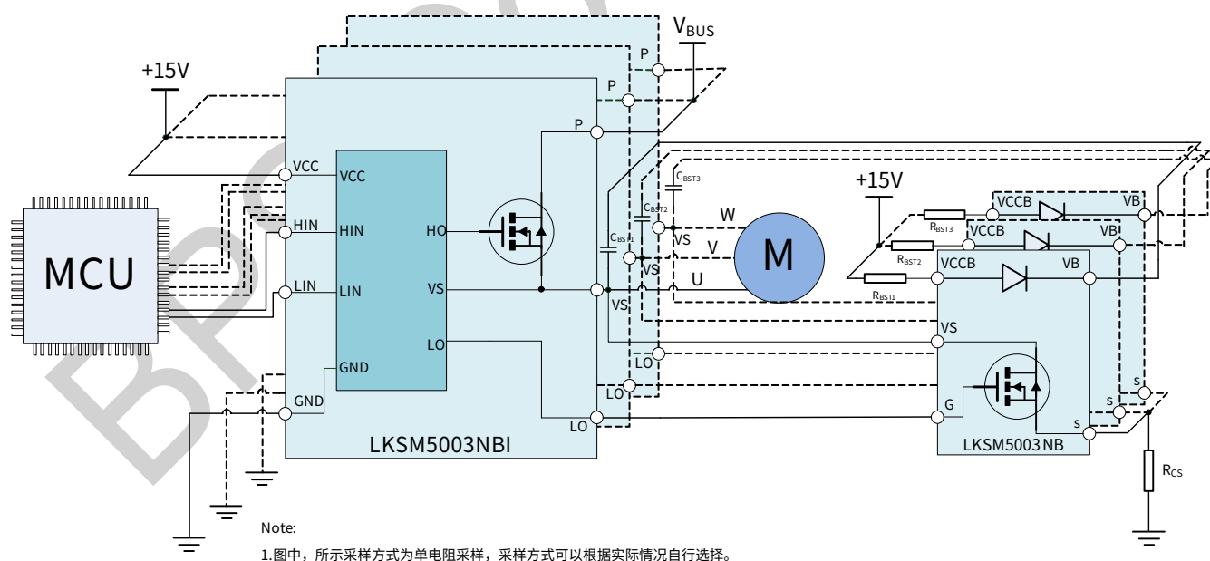
图 1. LKSM5003NBI & LKSM5003NB 典型应用图
