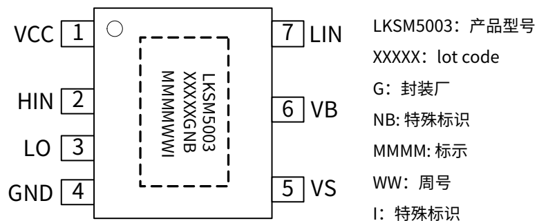
图 2. LKSM5003NBI 管脚封装图
