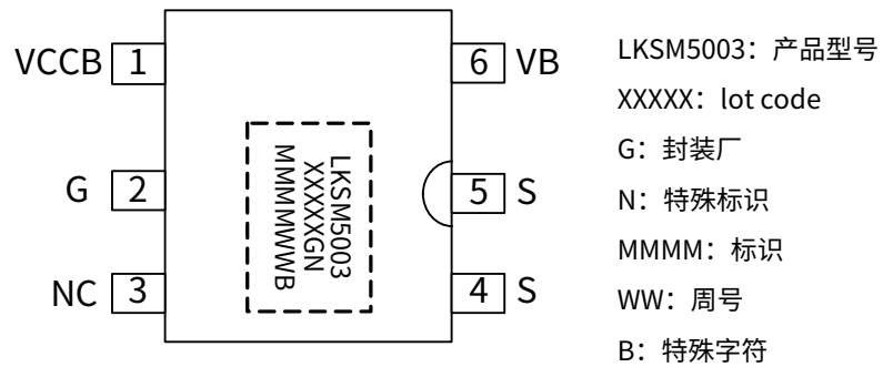
图 3. LKSM5003NB 管脚封装图
