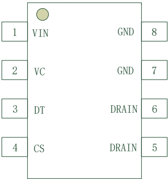
图 2-1 LKS610 管脚分布图
