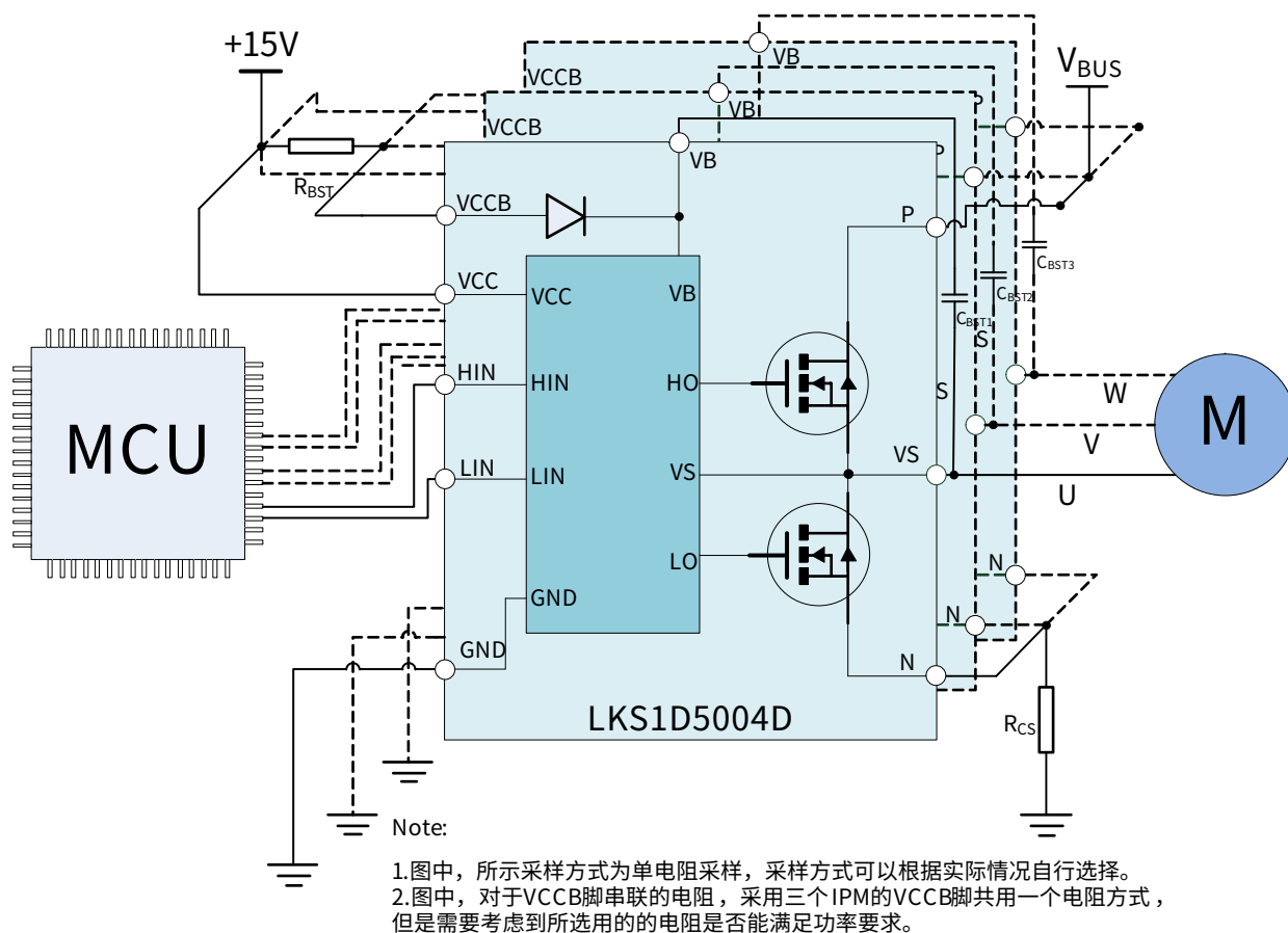
图 1. LKS1D5004D 典型应用图
