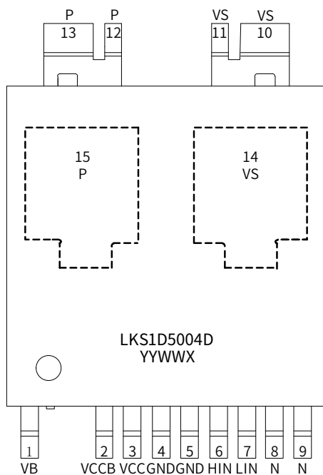
图 2. LKS1D5004D 管脚封装图
