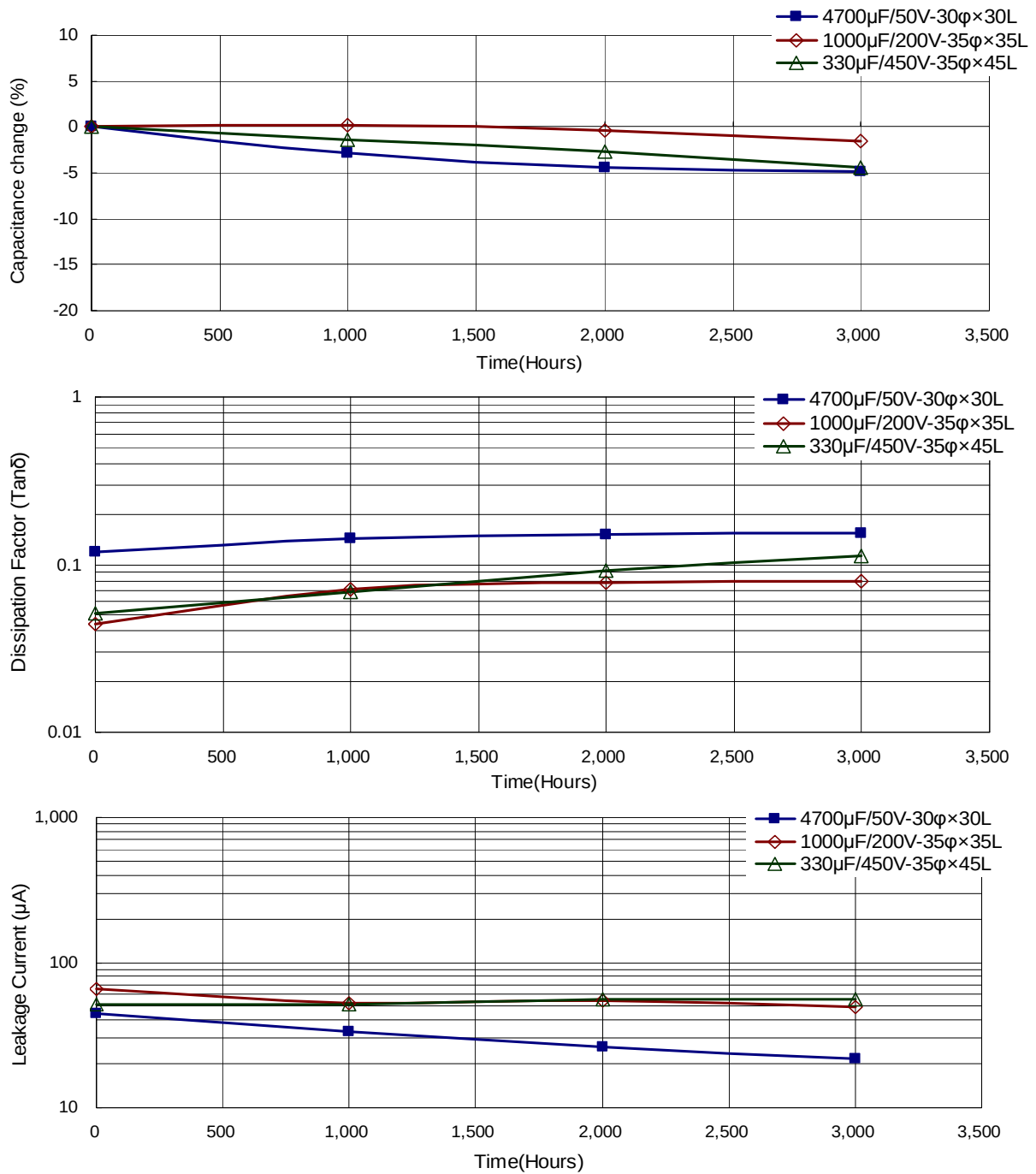
使用寿命图
