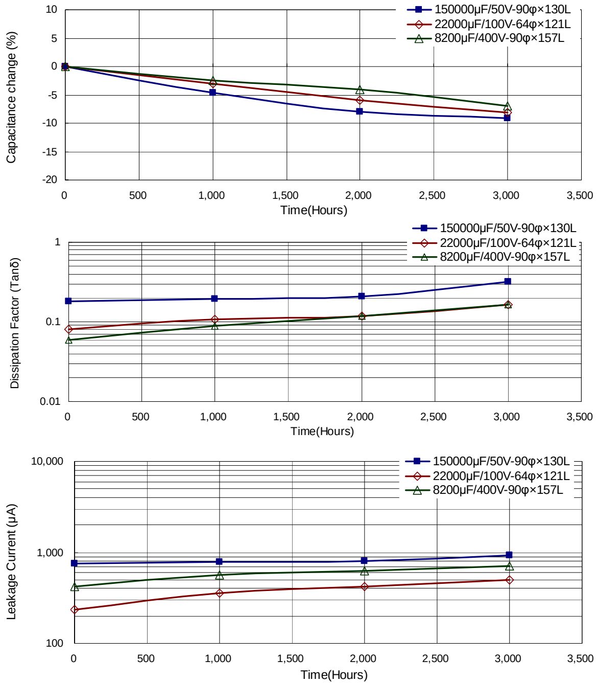
使用寿命图
