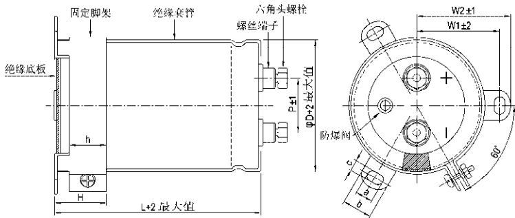
寸法图
