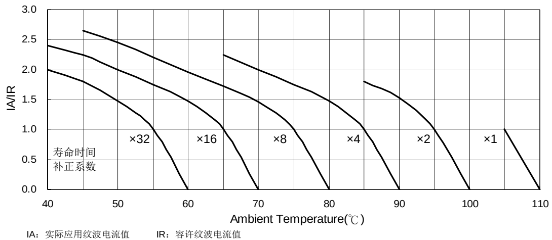
使用寿命图
