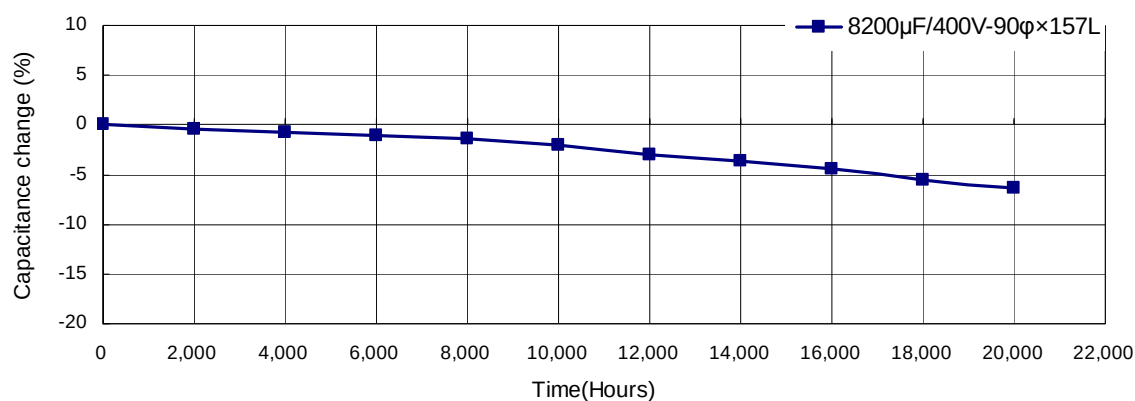
耐久性曲线
